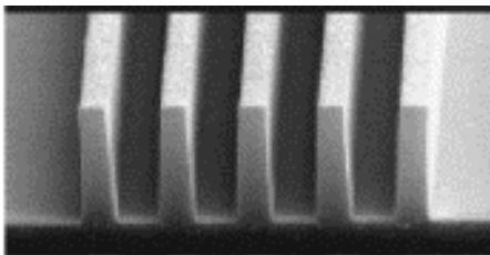
Рис. 2. Толщина линий 1 мкм, расстояние между линиями 1 мкм, высота линий 3 мкм
